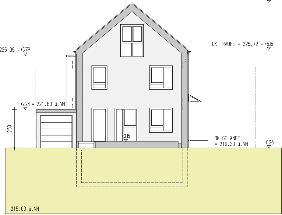
ANSICHT SUD
