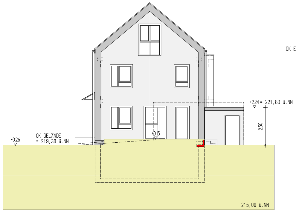
ANSICHT NORD
